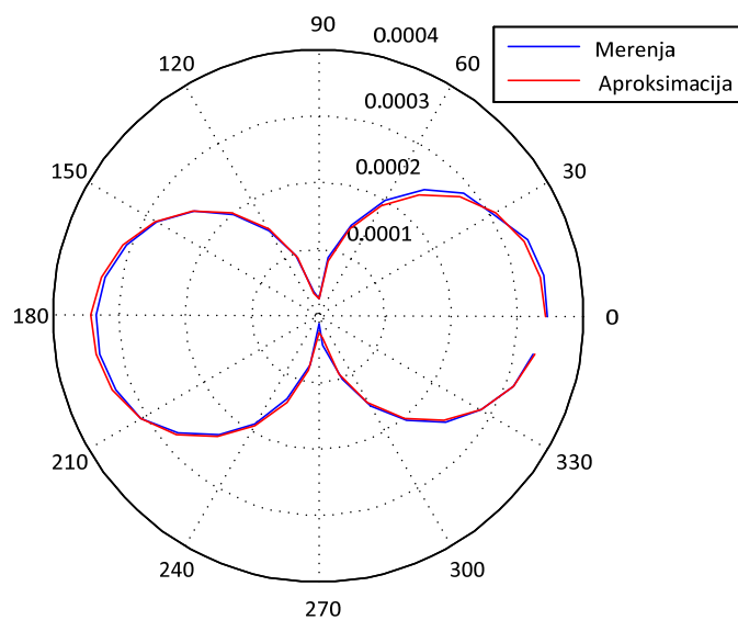
Slika 5.20 Uporedni polarni prikaz efektivne vrednosti struje druge serije merenja na konektoru prijemne antene i aproksimirane struje koju dominantni ekvivalentni dipol, postavljen paralelno x-osi, indukuje na pristupu prijemne antene, predajna antena je postavljena horizontalno, prijemna antena je horizontalni monopol, za f = 150 MHz
